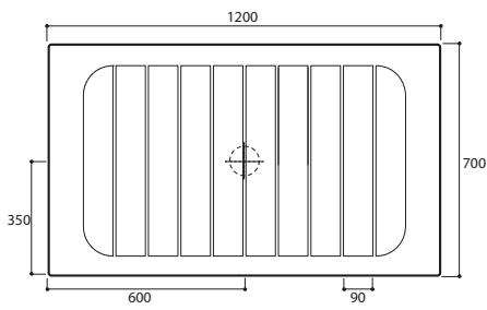
art. FL 12070
