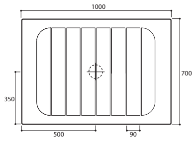
art. FL 10070
