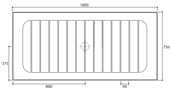
art. FL 16075
