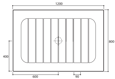
art. FL 12080
