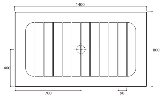
art. FL 14080
