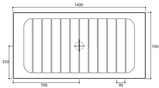
art. FL 14070
