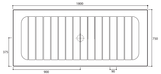
art. FL 18075
