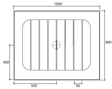
art. FL 10080
